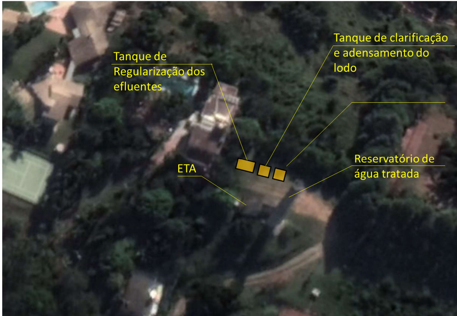
Figura 17 ETA II Layout preliminar de implantação do sistema de tratamento dos efluentes
